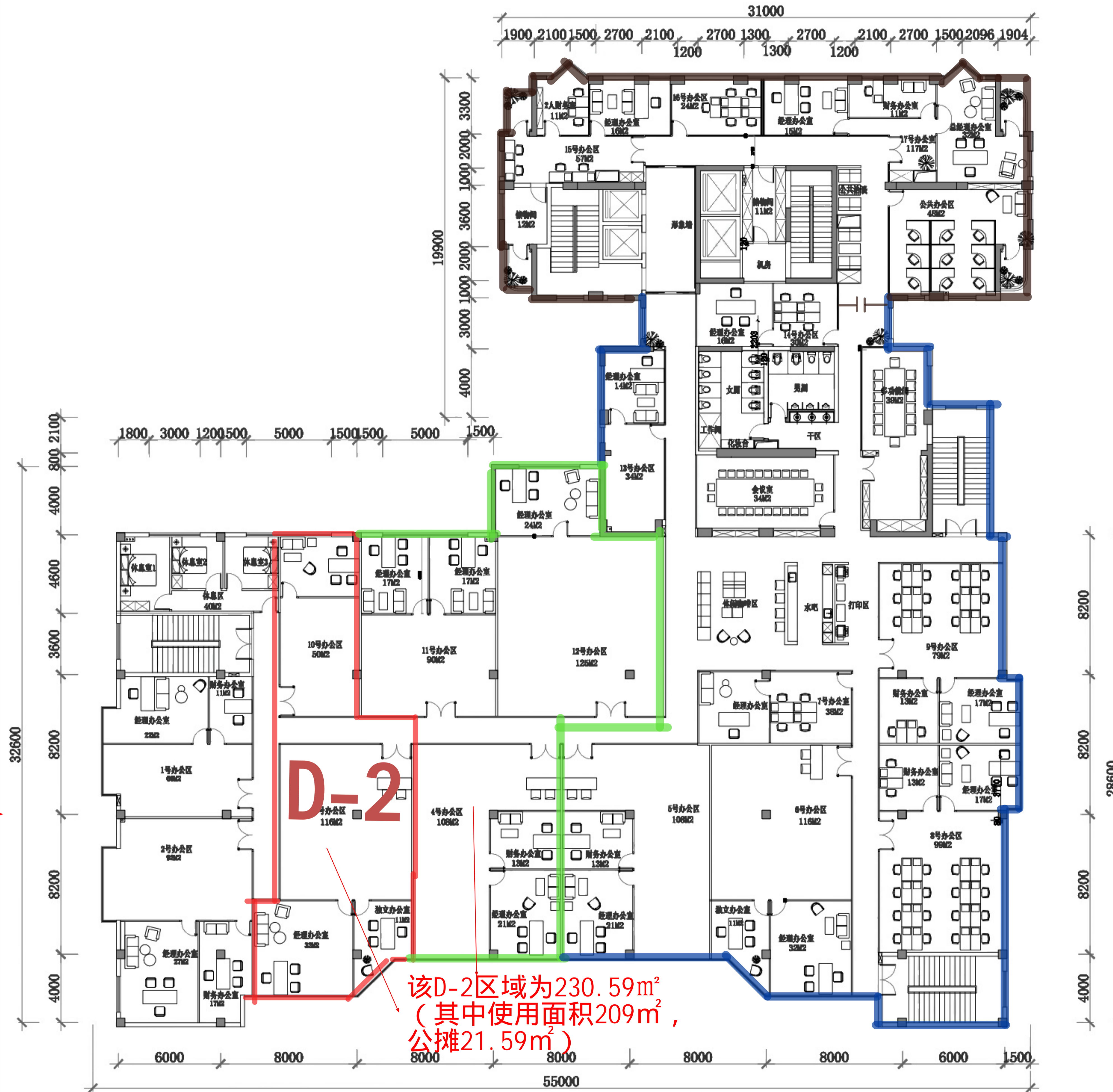
五层平面布置图 产权为2192.01平方米=使用(484+415+360+727)+公摊206.01
