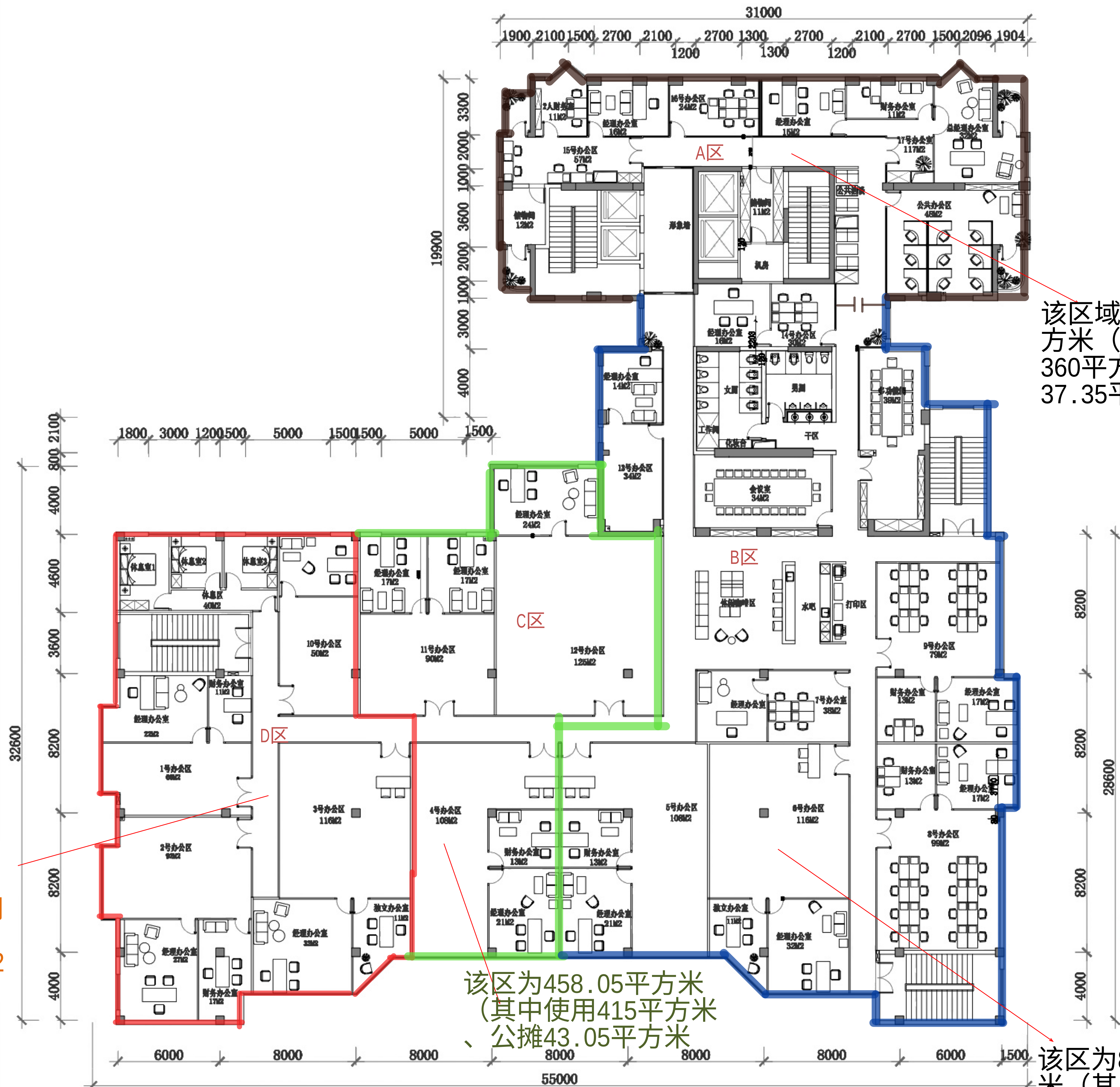
五层平面布置图 产权为2192.01平方米=使用（484+415+350+727）+公摊206.01
